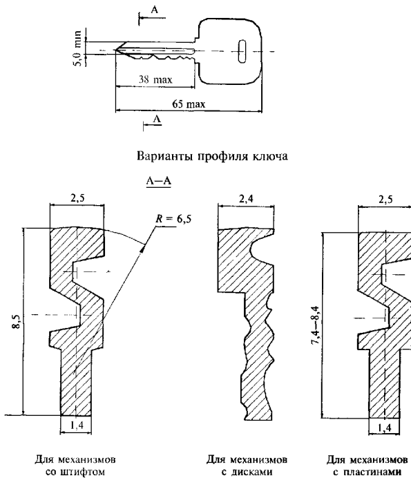
Рисунок В.44 — Пример ключа для цилиндрического механизма с односторонней нарезкой секретов
