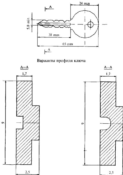
Рисунок В.45 — Пример ключа для цилиндрического механизма с двухсторонней нарезкой секретов
