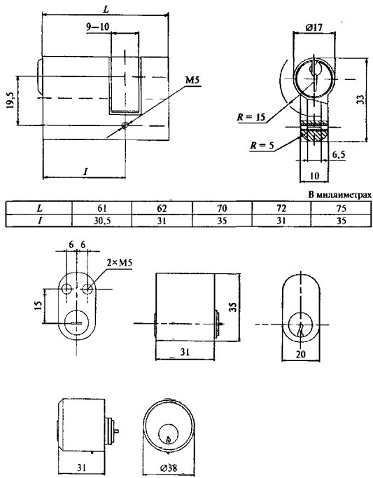
Рисунок В.25 — Примеры механизмов цилиндрических односторонних для врезных замков, тип МЦ3
