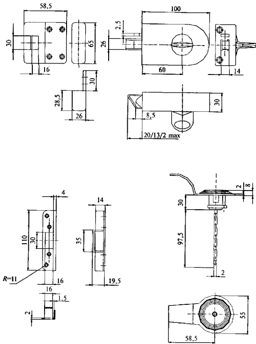
Рисунок В.17 — Пример замка накладного цилиндрического типа ЗН2 с автоматическим выводом засова-защелки
