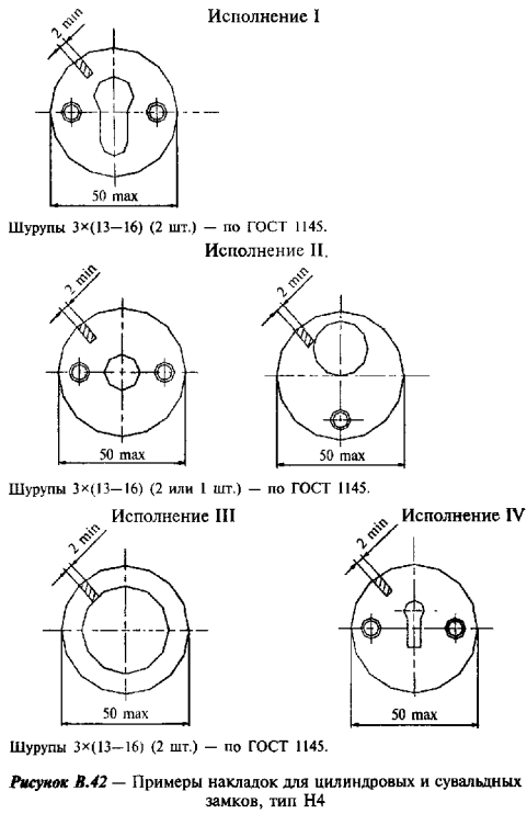
"Рис. В.42. Примеры накладок для цилиндрических и сувальдных замков, тип Н4"
