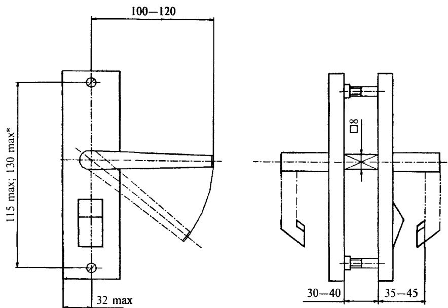
Рисунок В.36 — Пример ручек фалевых с накладками для защелок, тип РФ5
