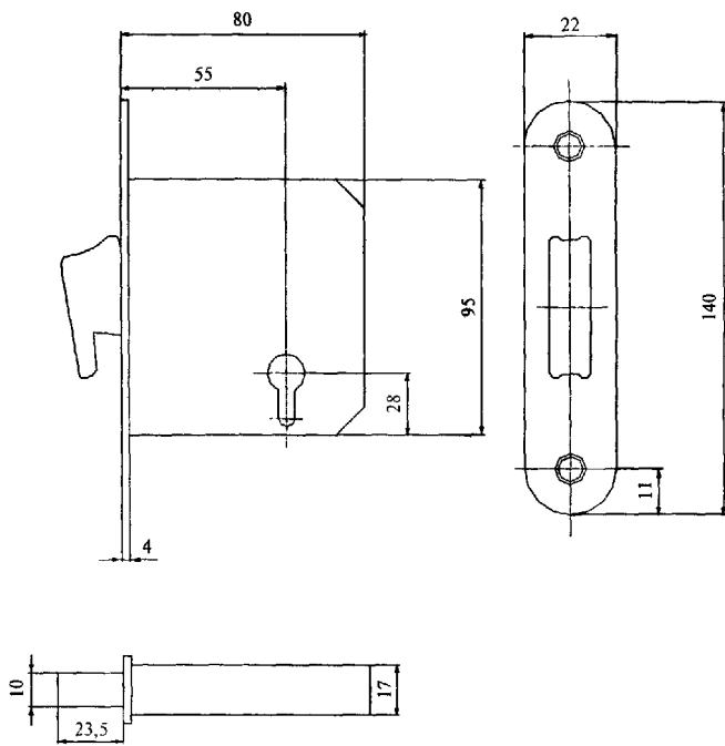
Рисунок В.2 — Пример замка врезного цилиндрического типа ЗВ1 с крюкообразным засовом
