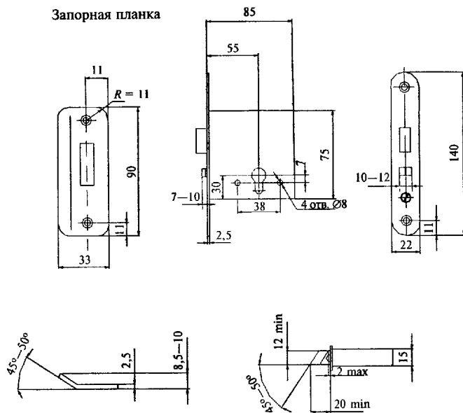
Рисунок В.5 — Пример замка врезного цилиндрического типа 3В2 с автоматическим выводом засова-защелки
