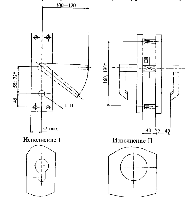
Рисунок В.32 — Пример ручек фалевых с накладками для замков, тип РФ1
