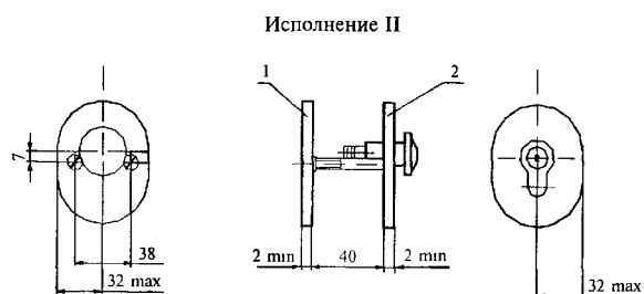
Рисунок В.38 — Пример накладок для врезных цилиндрических замков, тип Н1
