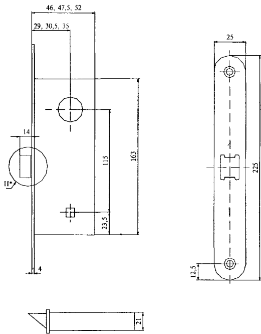
Рисунок В.11 — Пример замка врезного цилиндрического типа 3B4 для дверных блоков из поливинилхлоридных или алюминиевых профильных деталей
