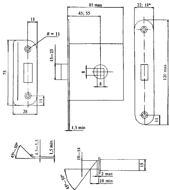
Рисунок В.19 — Пример защелки врезной типов ЗЩ1 и ЗЩ1Д
