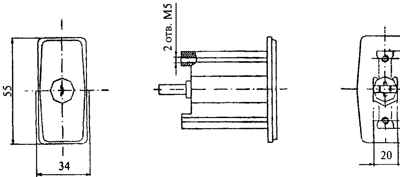
Рисунок В.31 — Пример механизма цилиндрического штифтового для врезных замков, тип МЦ11
