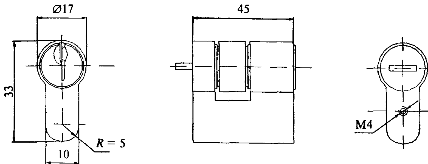
Рисунок В.28 — Пример механизма цилиндрического пластинчатого для накладных замков, тип МЦ8
