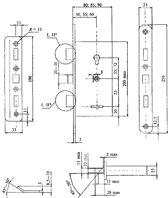
Рисунок В.14 - Пример замка врезного комбинированного с цилиндрическим и сувальдным механизмами секретности и защелкой типа ЗВ13
