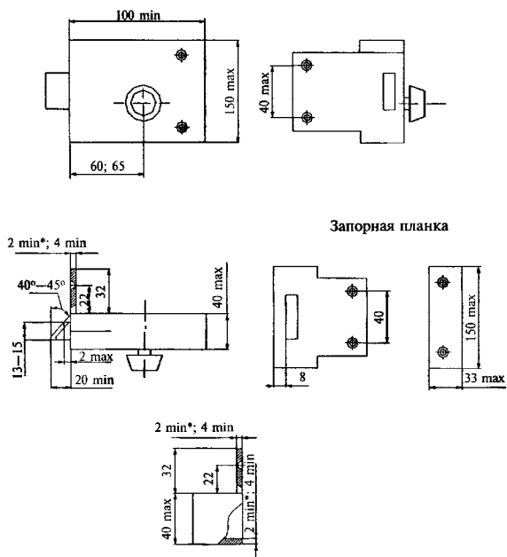
"Рис. В.15. Пример замка накладного цилиндрического (тип ЗН1) и сувальдного (тип ЗН4)"
