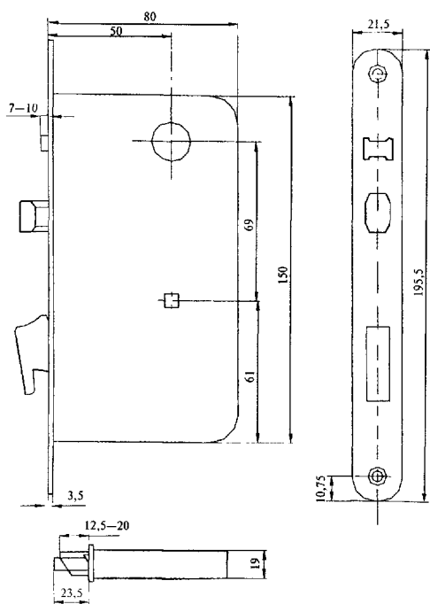
Рисунок В.8 — Пример замка врезного цилиндрического типа ЗВ7 с крюкообразным засовом и автоматическим выводом засова-защелки
