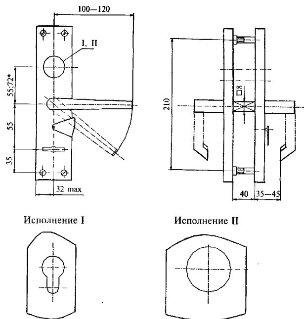
Рисунок В.34 — Пример ручек фалевых с накладками для замков, тип РФ3
