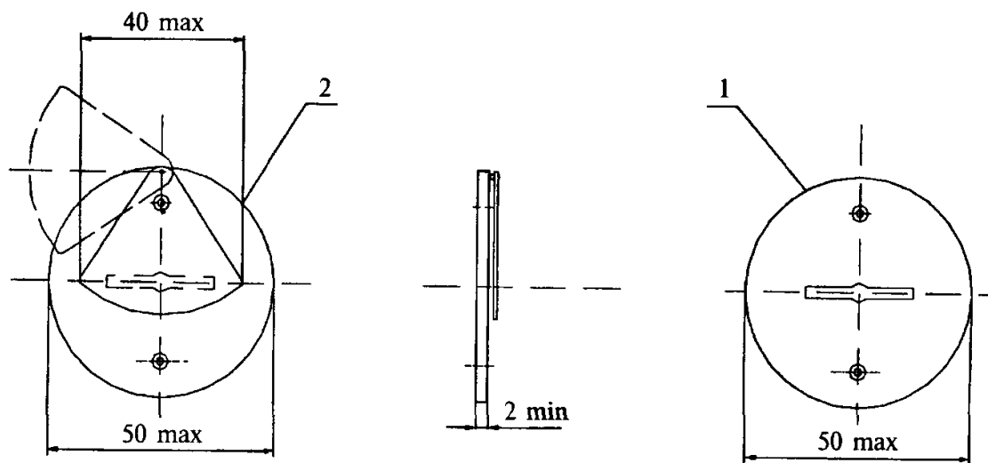
"Рис. В.39. Пример накладок для врезных замков с цилиндрическим механизмом МЦ4, тип Н2"
