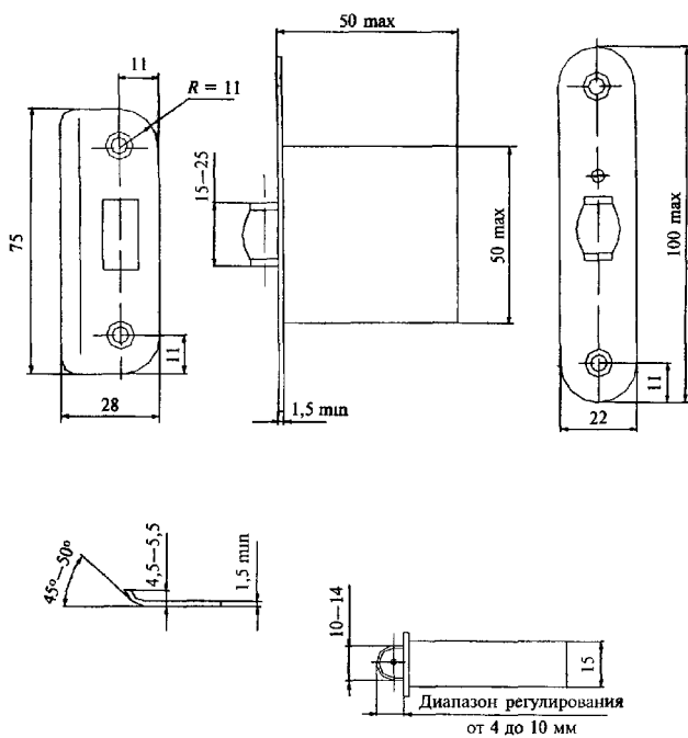
Рисунок В.22 — Пример защелки врезной типа ЗШ4
