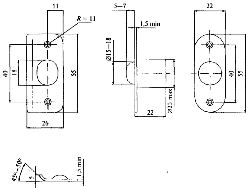
Рисунок В.21 — Пример защелки врезной типа ЗШЗ
