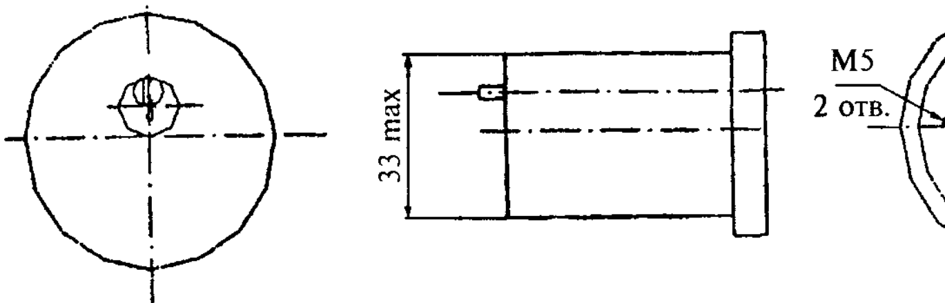
Рисунок В.30 — Пример механизма цилиндрического штифтового для накладных замков, тип МЦ10
