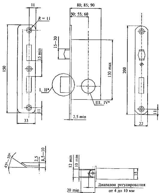
Рисунок В.13 - Пример замка врезного цилиндрического (типы ЗВ5) или сувальдного (ЗВ10) с прямым засовом и роликом
