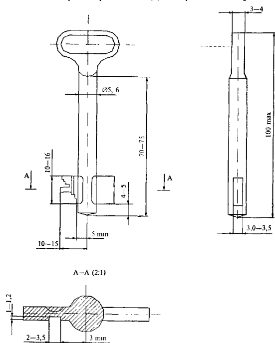
Рисунок В.47 — Пример ключа для накладного сувальдного замка, тип ЗС2
