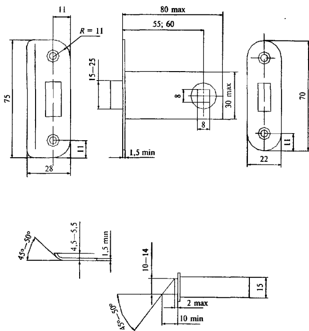
"Рис. В.19. Пример защелки врезной типов ЗЩ1 и ЗЩ1Д"
