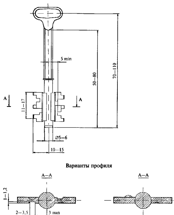
Рисунок В.46 — Пример ключа для врезного сувальдного замка, тип ЗС1
