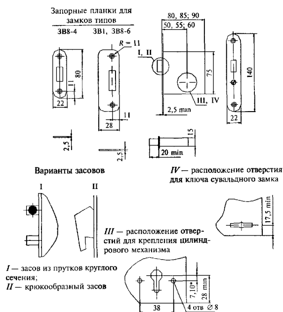
Рисунок В.1 — Пример замка врезного цилиндрического (тип 3В1) или сувальдного (тип 3В8)
