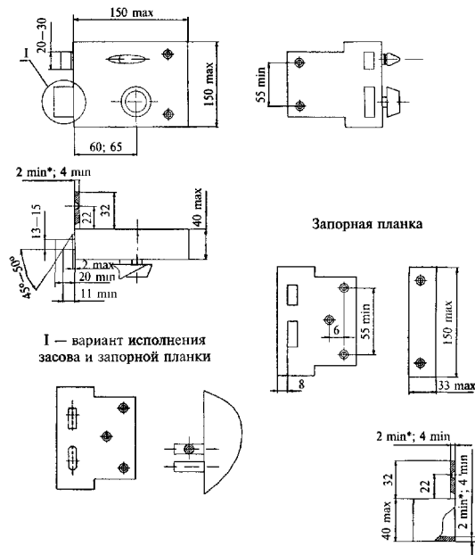
"Рис. В.17. Пример замка накладного цилиндрического типа ЗН2 с автоматическим выводом засова-защелки"
