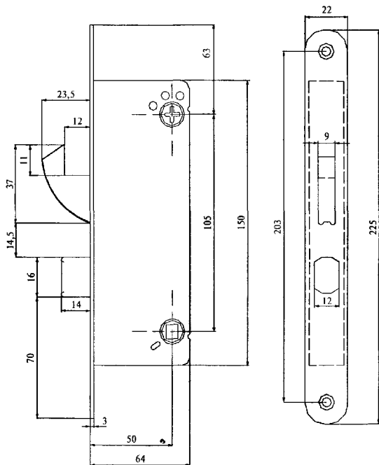
Рисунок В.12 — Пример замка врезного цилиндрического типа 3B7 с защелкой и крюкообразным засовом для дверных блоков из поливинилхлоридных или алюминиевых деталей
