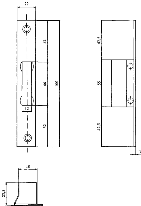
"Рис. В.42. Примеры накладок для цилиндрических и сувальдных замков, тип Н4"
