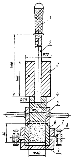
1—рукоятка; 2—направляющий стержень; 3—цилиндр; 4—плунжер; 5—направляющий насадный цилиндр; 6—разъемный цилиндр; 7—подставка; 8—закрепляющие винты; 9—металлическая пластинка
