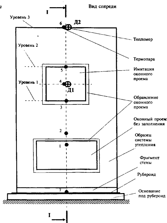
Рисунок 2 — Схема установки с образцом системы утепления
