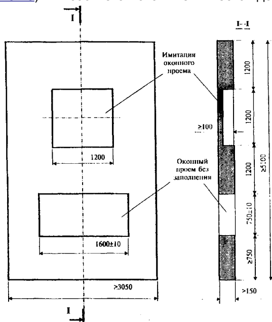
Рисунок 1 - Фрагмент стены
