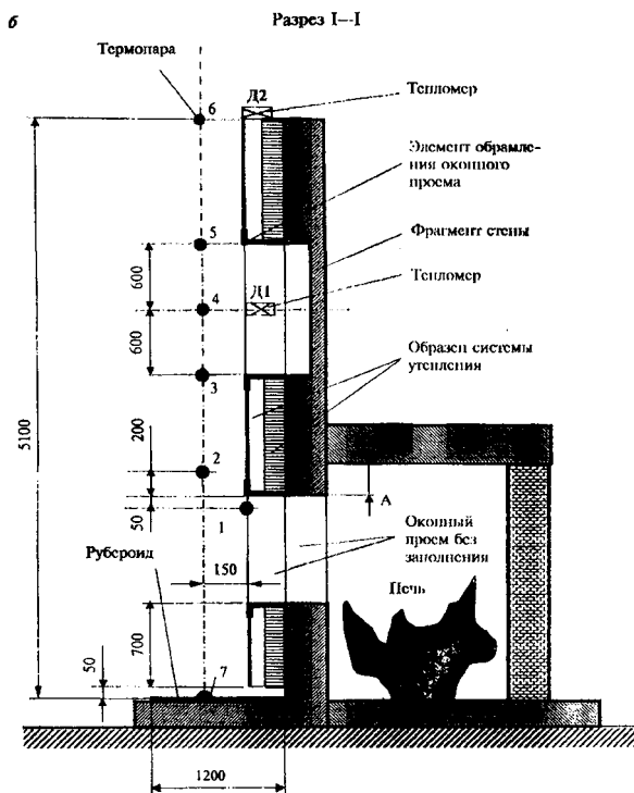
"Рисунок 2б. Схема установки с образцом системы утепления (разрез)"
