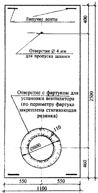
"Рис. 1. Элементы раздвижной деревянной рамы"
