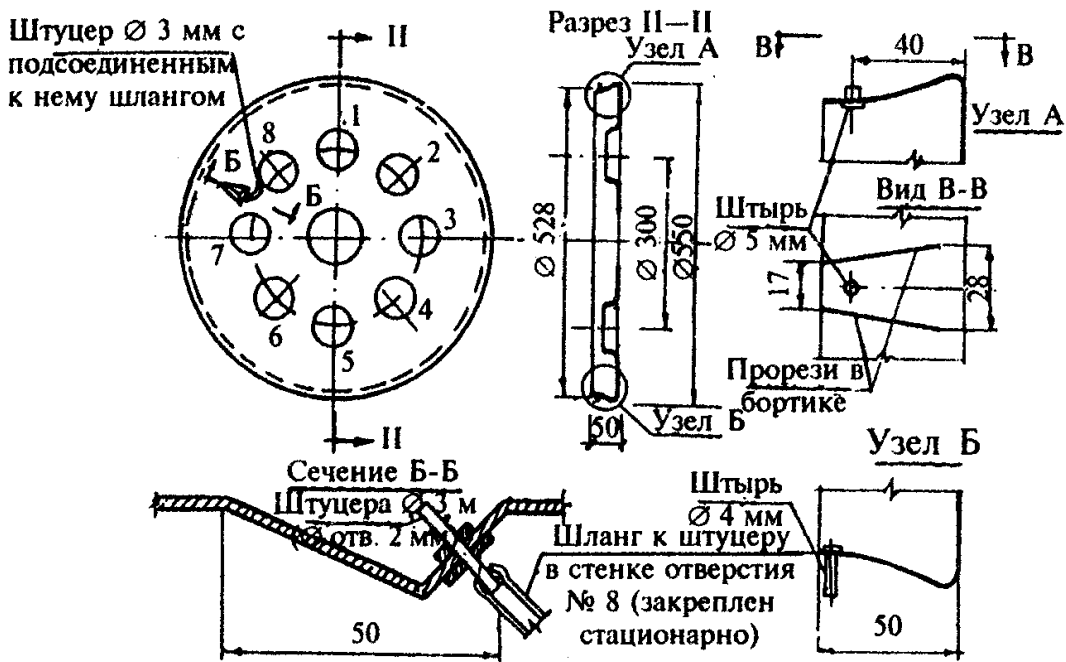
"Рис. 3. Кожух вентилятора"
