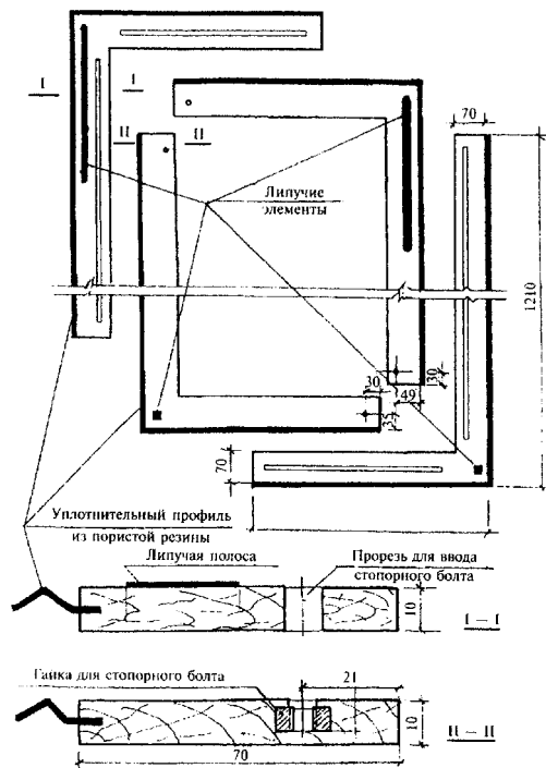
Рисунок 1 — Элементы раздвижной деревянной рамы
