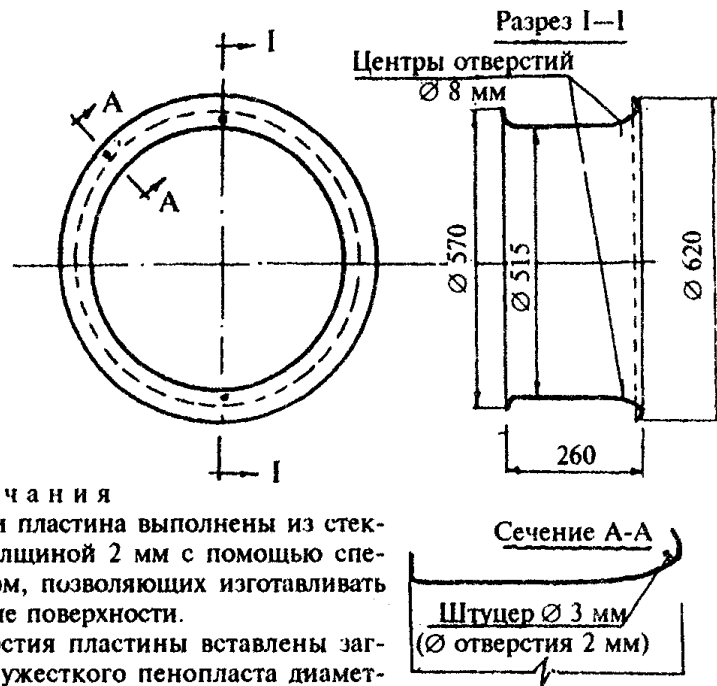
Рисунок 3 — Кожух вентилятора
