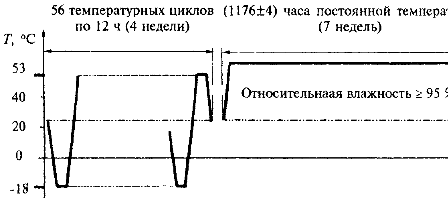
Рисунок А.1 — График испытаний стеклопакетов по режиму
