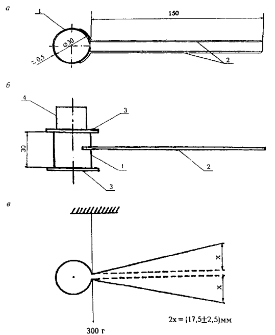
а — кольцо Ле Шателье (вид сверху); б — кольцо Ле Шателье с пластинками и пригрузом (вид сбоку); в — схема проверки упругости кольца Ле Шателье 1 — кольцо с прорезью; 2 — индикаторная игла; 3 — пластинка; 4 — пригруз
