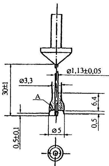
Рисунок 5 — Рабочая часть короткой иглы с кольцеобразной насадкой
