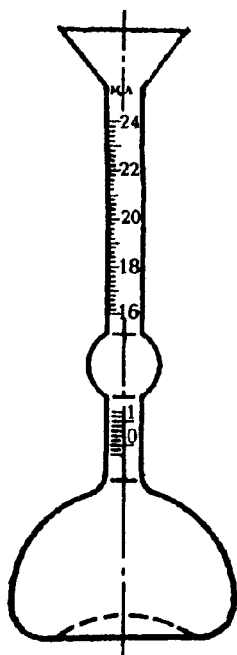
Рисунок 1 — Прибор Ле Шателье
