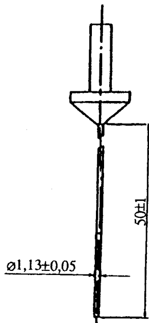
Рисунок 4 — Рабочая часть длинной иглы
