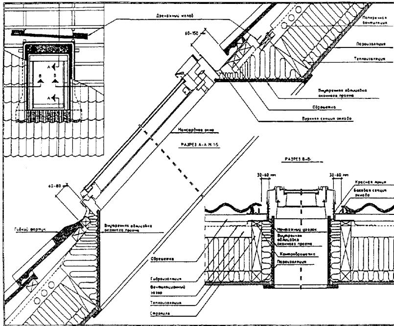
Рисунок А.2 — Пример конструкции монтажного узла
