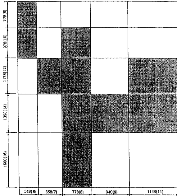
Рисунок 2 — Рекомендуемые габаритные размеры мансардных оконных блоков (мм)
