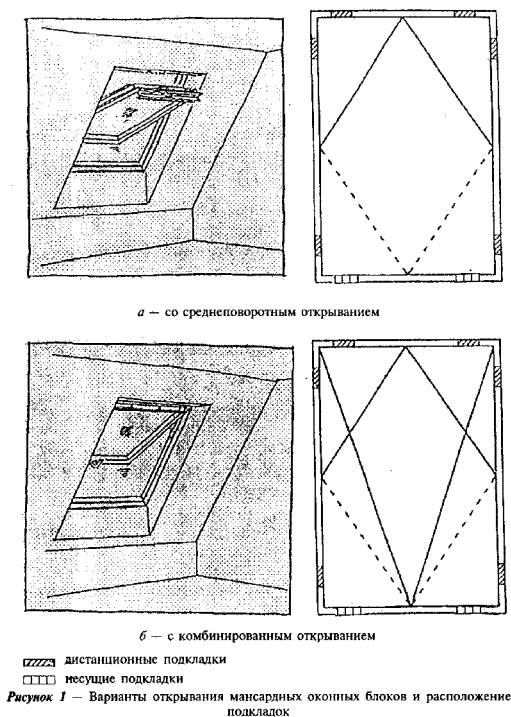
"Рис. 1. Варианты открывания мансардных оконных блоков и расположение подкладок"
