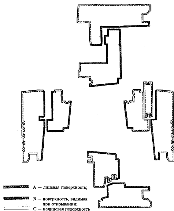
Рисунок 4 – Виды поверхностей деталей
