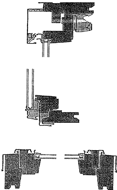
Рисунок 3 — Пример конструктивного решения мансардного оконного блока
