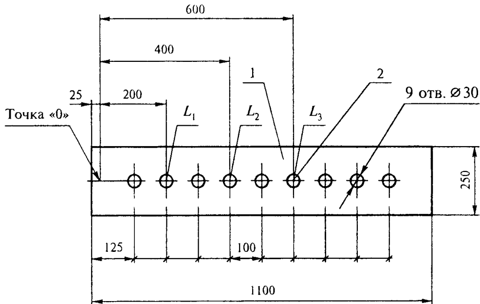
Рисунок 4 — Калибровочный образец
