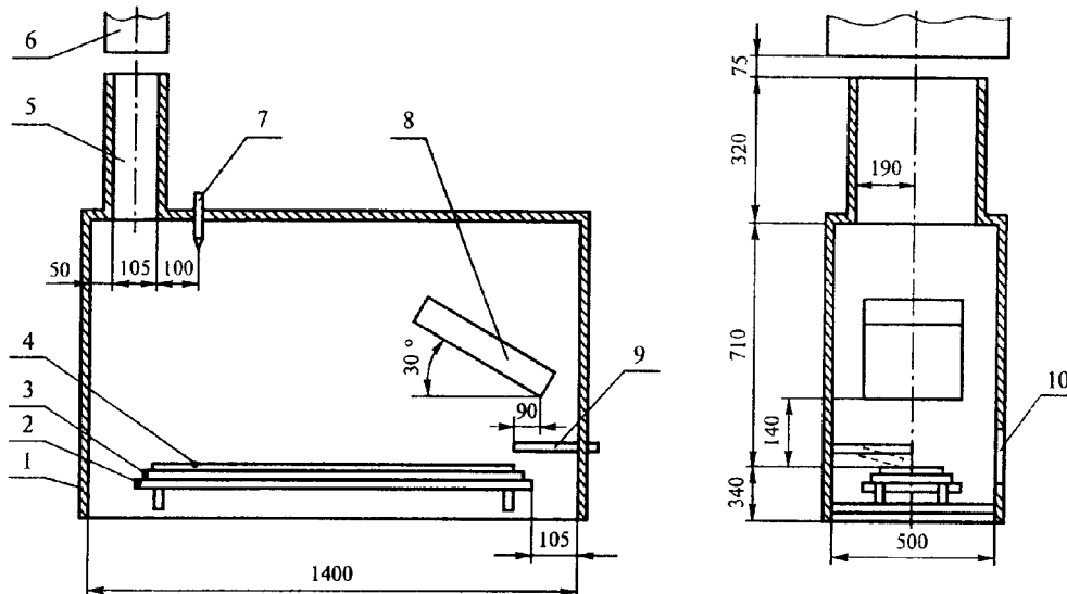
1 — испытательная камера; 2 — платформа; 3 — держатель образца; 4 — образец; 5 — дымоход; 6 — вытяжной зонт; 7 — термопара; 8 — радиационная панель; 9 — газовая горелка; 10 — дверца со смотровым окном
