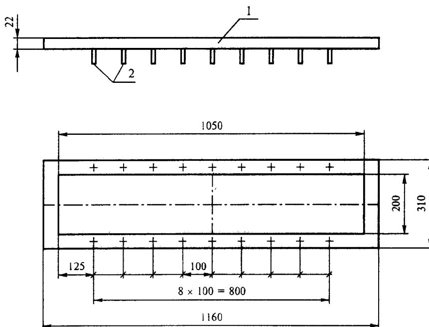
Рисунок 3 — Держатель образца
