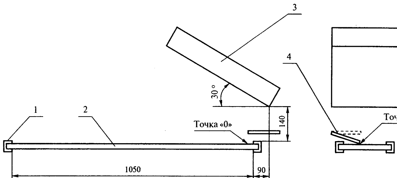
1 — держатель; 2 — образец; 3 — радиационная панель; 4 — газовая горелка
