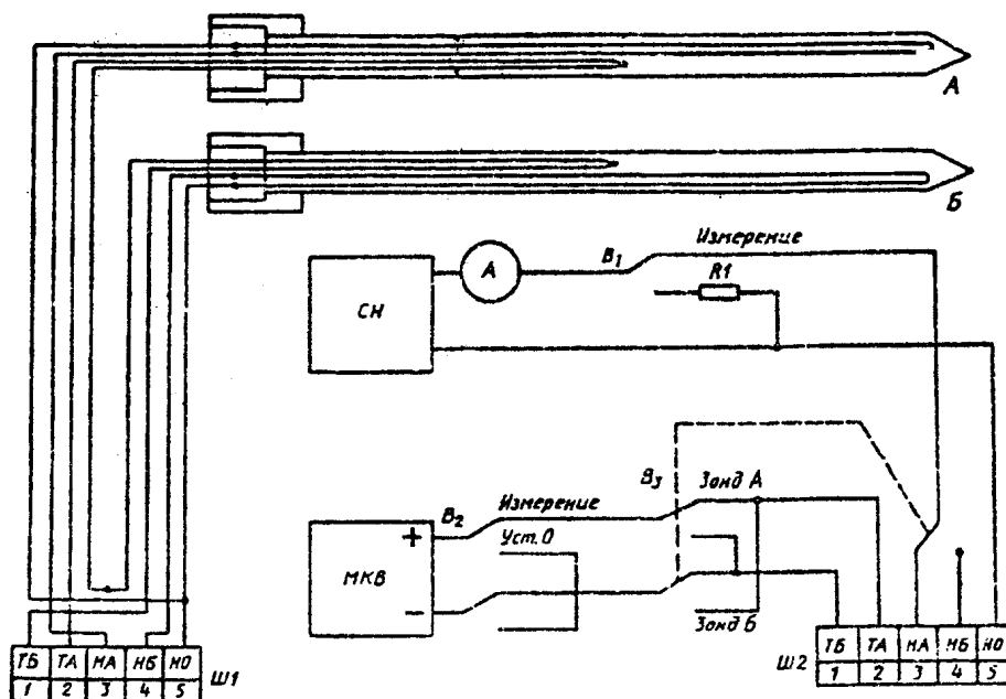
Рисунок 1 — Устройство зонда и электрическая схема соединения приборов
