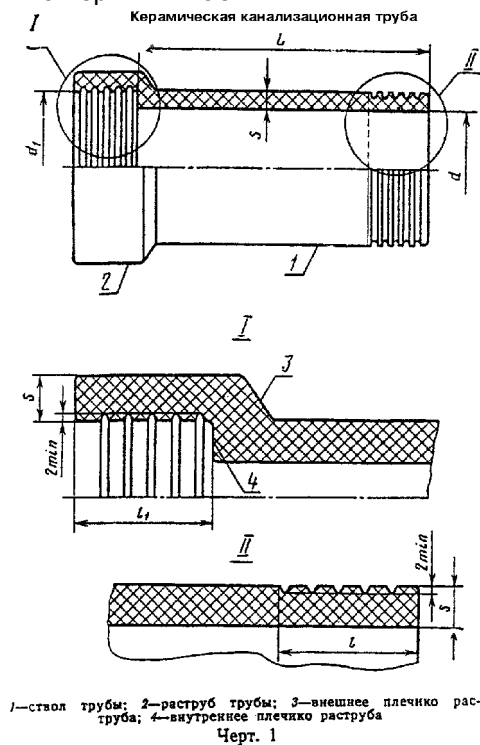
"Чертеж 1. Керамическая канализационная труба"
