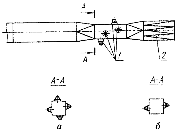
a — четыре громкоговорителя; б — два громкоговорителя; 1 — громкоговорители; 2 — концевое поглощающее устройство
