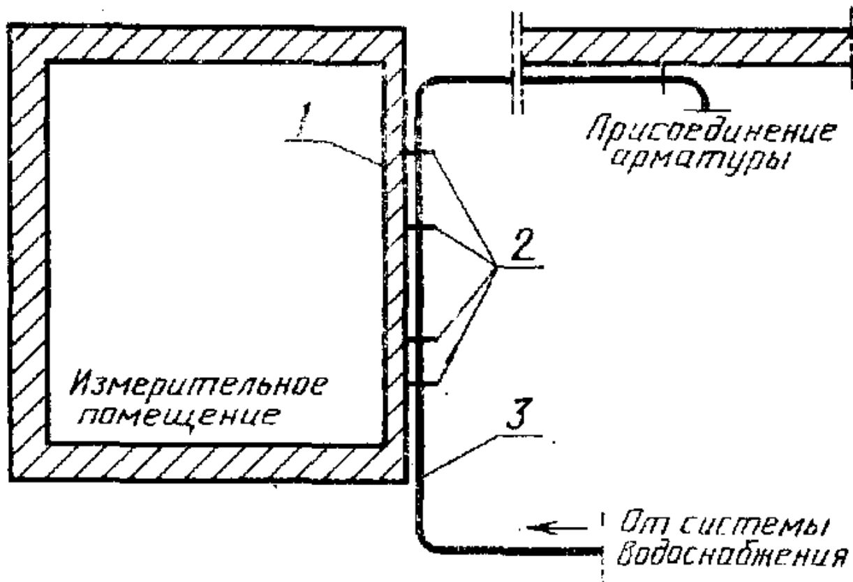
1—испытательная стена; 2—кронштейны; 3—испытательный трубопровод Черт. 3
