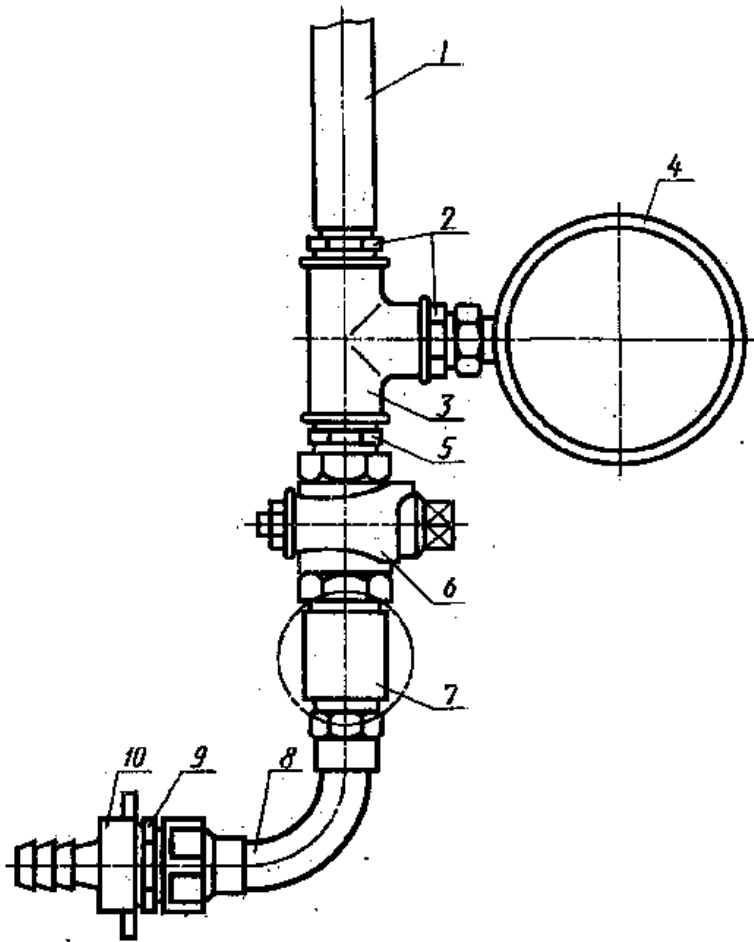
1—провод 3/4"; 2—диффузор 3/4"-1; 3—тройник 1"; 4—манометр; 5—ниппель 1"; 6—шариковый кран; 7—ЭГШ; 8—колено; 9—ниппель 3/4"; 10—выход воды
