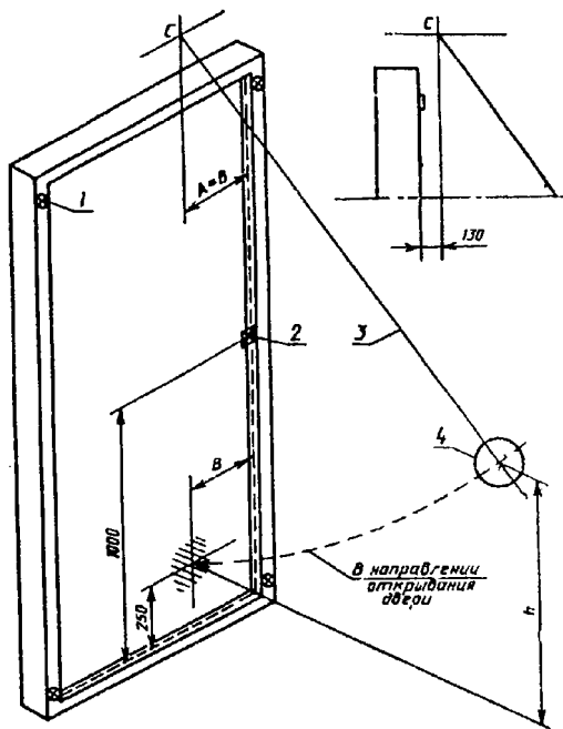
1 — пружин; 2 — запирающий прибор или ограничитель; 3 — гибкая нить; 4 — неупругое тело (груз). B — 1/2 ширины полотна, но не более 300 мм.
