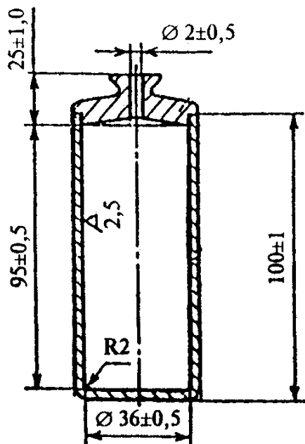
Рисунок 3 — Пикнометр
