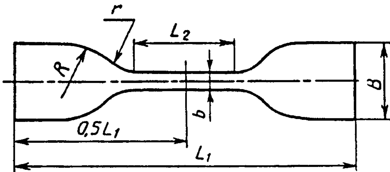
Рисунок 2 — Образец-лопатка типа 2
