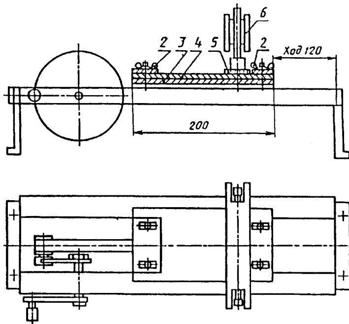
1 — рукоятка; 2 — зажимные винты; 3 — пластинка; 4 — образец; 5 — щетка; 6 — груз Рисунок 7
