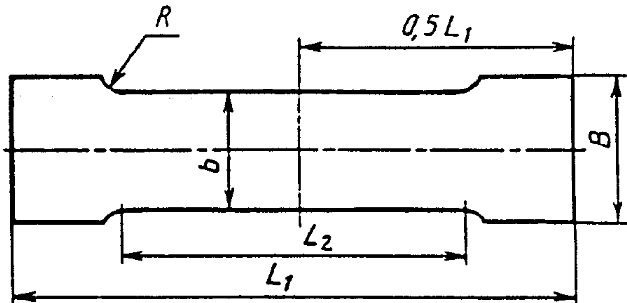
Рисунок 1 — Образец-лопатка типа 1
