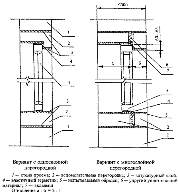
Рисунок 1 — Схема проема испытательной камеры со вспомогательной перегородкой
