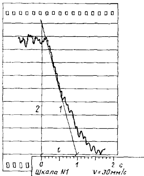
"Пример оценки реверберационной кривой"
