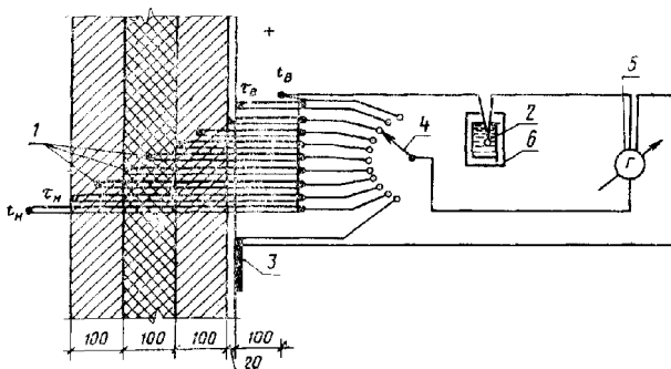
Сечение стёны и подключение датчиков
