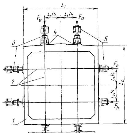
1—звено трубы; 2—металлические тяжи; 3—гидродомкраты; 4—слой цементно-песчаного раствора; 5—металлические траверсы; 6—опоры; F_v —вертикальная нагрузка; F_h —горизонтальная нагрузка
