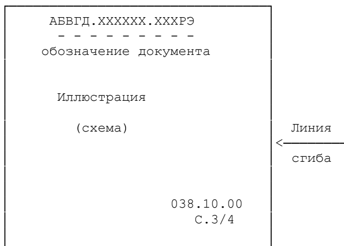
Рисунок Б.1 - Пример оформления листов увеличенного формата (правила фальцования)
