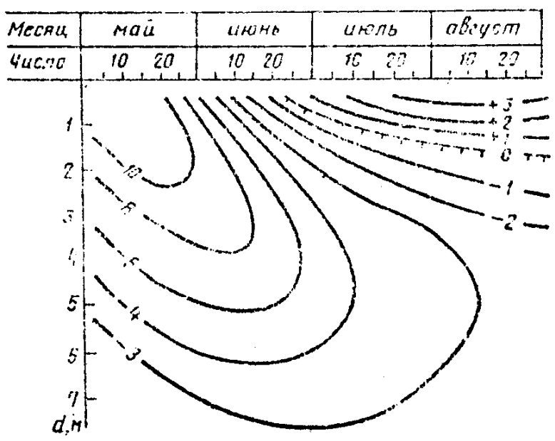
"График термоизоплент по данным режимных (длительных) температурных наблюдений"
