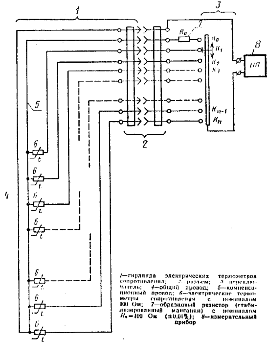
"Принципиальная схема подключения гирлянды термодатчиков к измерительному прибору"
