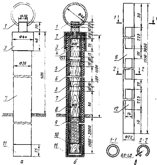
Мерзлотомер Ратомского
