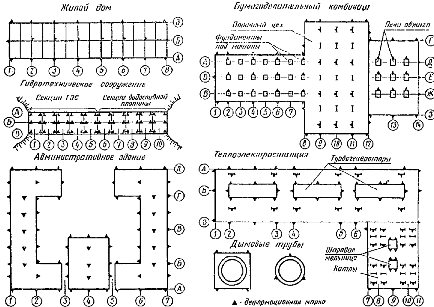
"Примеры расположения деформированных марок на зданиях и сооружениях"
