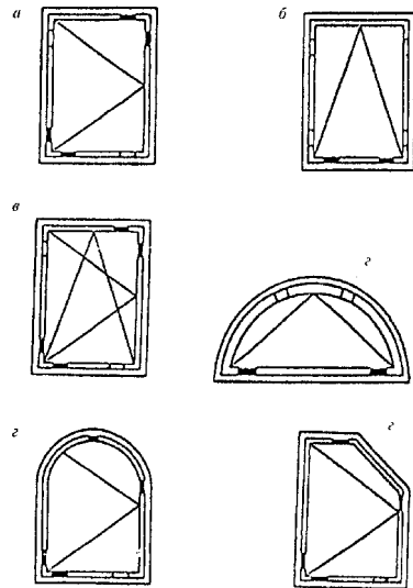
Виды открывания оконных блоков: a – поворотное (распашное); б – откидное; в – поворотно-откидное; г – установка подкладок в фигурных оконных блоках
