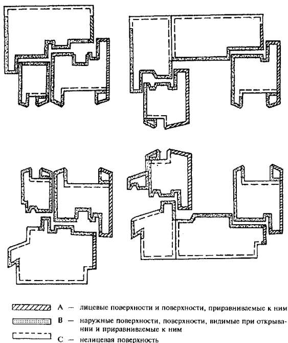
Рисунок 8 — Примеры определения видов поверхностей деталей
