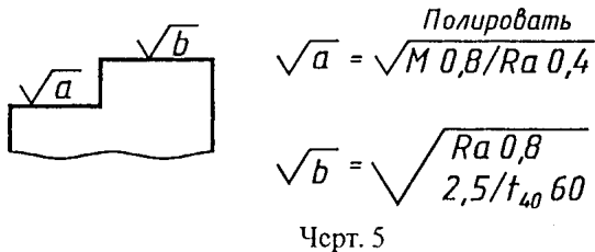
"Черт. 5 Упрощенное обозначение шероховатости поверхностей с его разъяснением"
