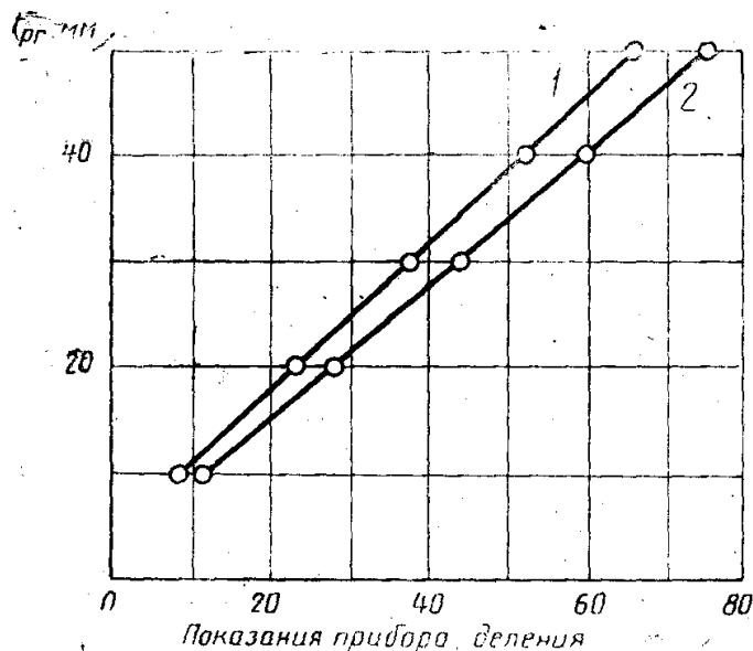
Чертеж В.1 — Градуировочные зависимости для продольных стержней диаметром 16 мм, 1 — при шаге стержней s=50 мм; 2 » » » » s=100 мм.
