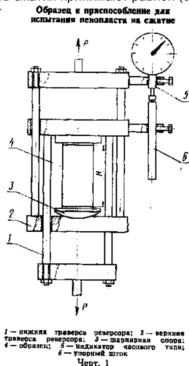
"Черт. 1. Образец и приспособление для испытания пенопласта на сжатие"
