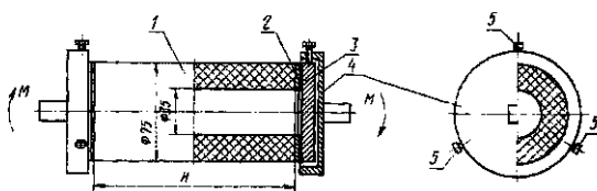
1 — образец; 2 — клей; 3 — опорная шайба; 4 — захватная муфта; 5 — зажимной винт Черт. 3
