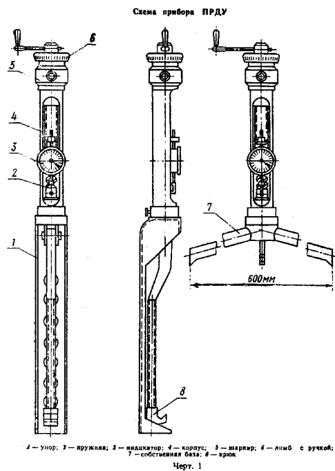
"Черт. 1. Схема установки прибора ПРДУ"
