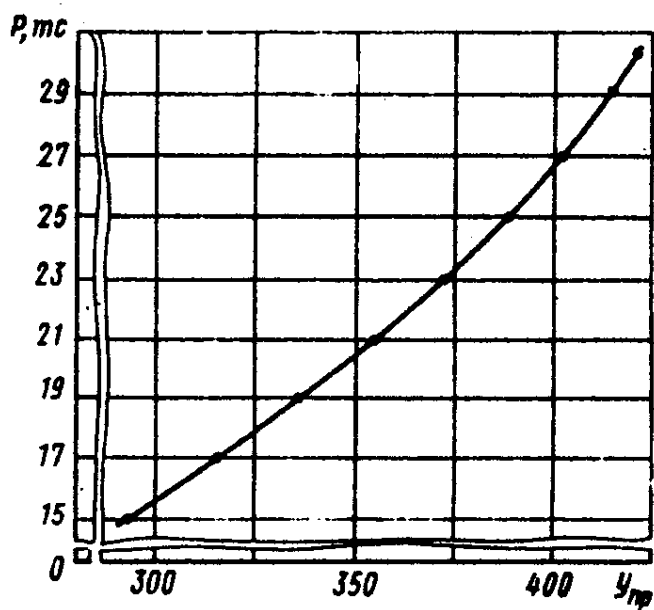
"Градуировочная характеристика прибора ПРДУ"
