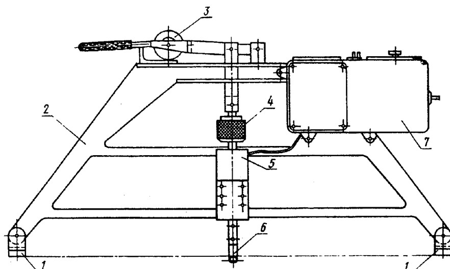
Схема прибора ПИН
