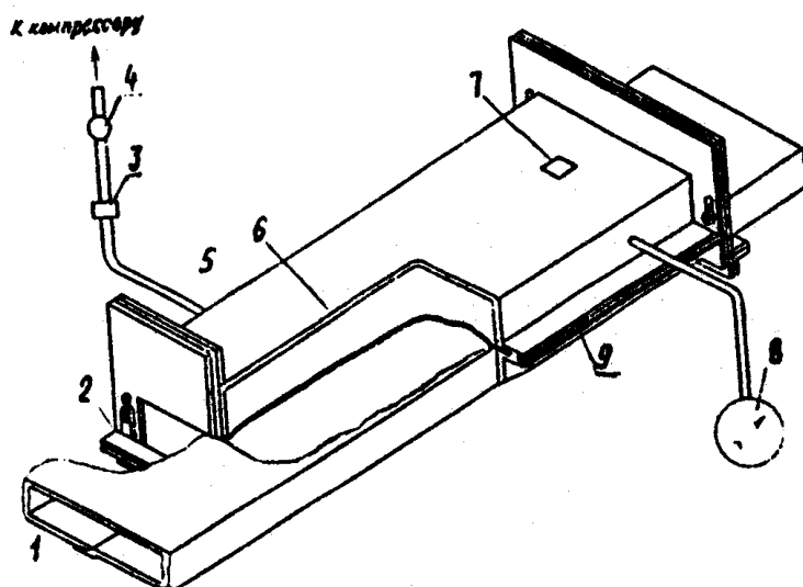
1-образец; 2-опора; 3-трехходовый кран; 4-вентиль; 5-короб; 6-резиновая мембрана; 7-предохранительный клапан; 8-манометр; 9-крепежные уголки
