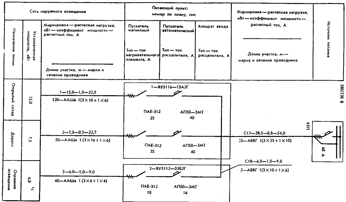
Черт. 2
