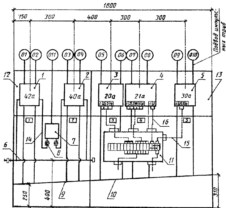
"Пример выполнения чертежа установки"
