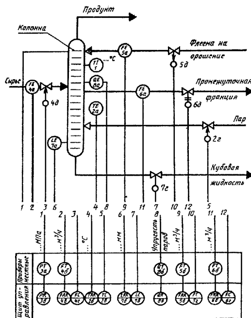
ПРИМЕР ВЫПОЛНЕНИЯ СХЕМЫ АВТОМАТИЗАЦИИ РАЗВЕРНУТЫМ СПОСОБОМ
