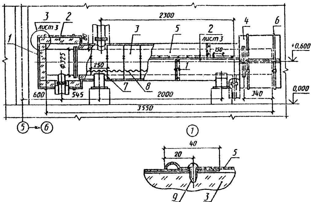
"Пример выполнения чертежа тепловой изоляции"
