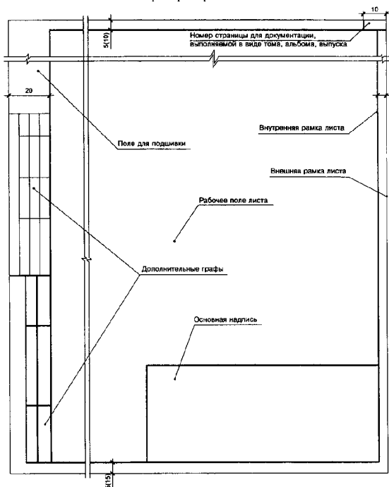
Расположение основной надписи, дополнительных граф к ней и размерных рамок на листах
