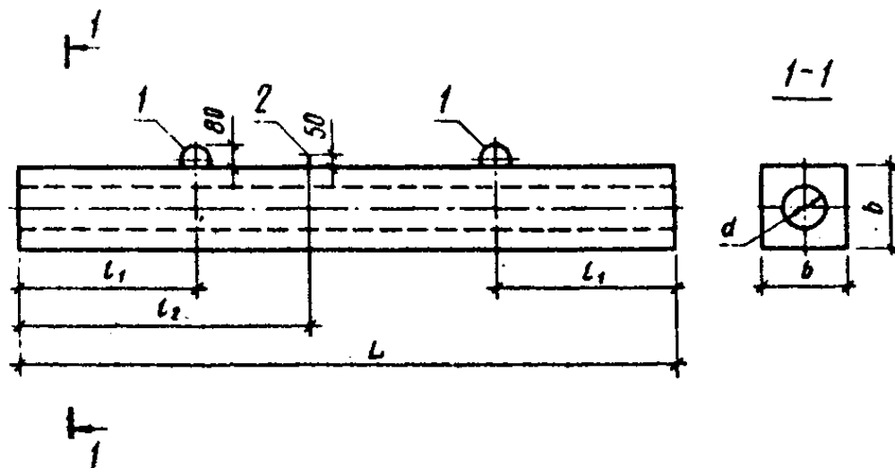
Сваи квадратного сечения с круглой полостью
