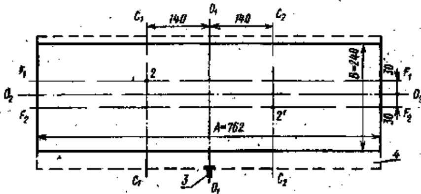
Схема расположения в рабочей камере АИП двух угольных дуговых ламп и зоны облучения
