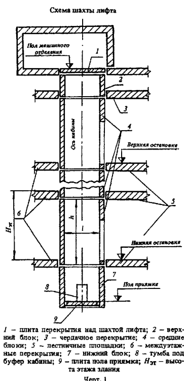
"Черт. 1. Схема шахты лифта"
