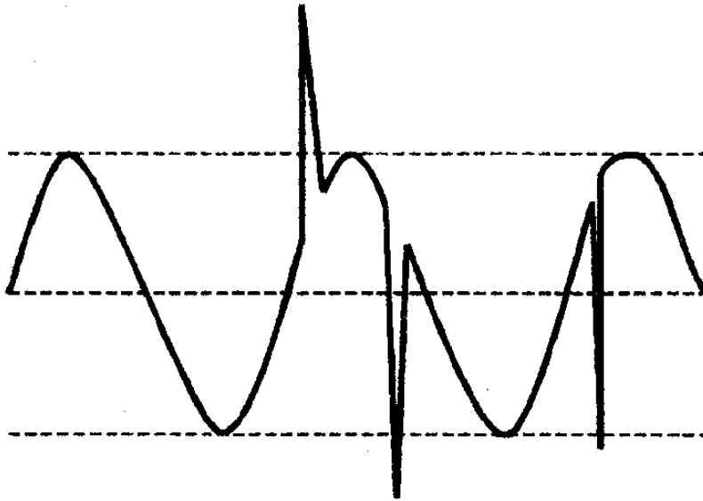
Рисунок А.3 — Импульсы напряжения
