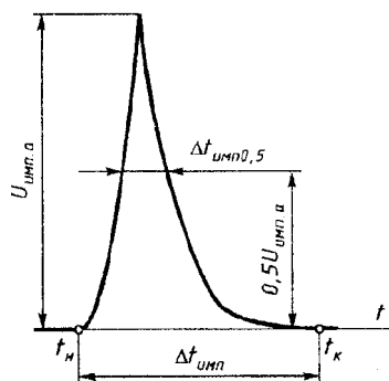
Рисунок Б.3 — Параметры импульсного напряжения
