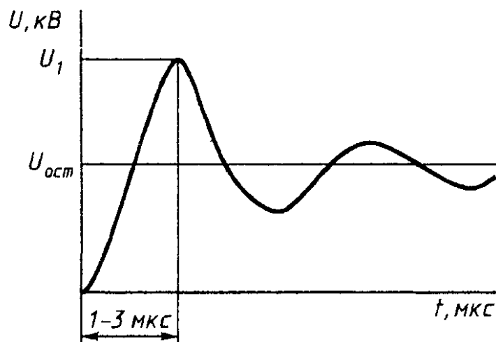
Рисунок Д.2 — Форма грозových импульсов, характерная для точек присоединения a , в , г , д на рисунке Д.1.
