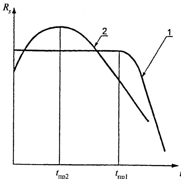
Рисунок 3 - Определение времени проникания t_{\text{пр}} агрессивных сред по различным видам записываемых потенциометром кривых изменения во времени поверхностного электрического сопротивления R_s
