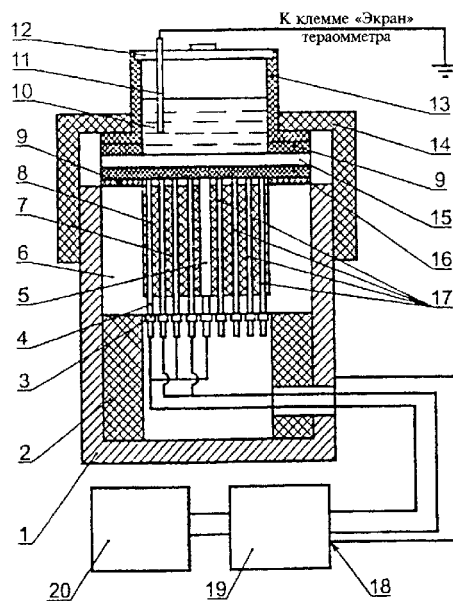
1 — корпус; 2 — подставка держателя; 3 — гайка крепления электродов; 4 — крепежный стержень электродов; 5 — центральный стержневой электрод; 6 — держатель кассеты; 7 — фторопластовая прокладка; 8 — кассета электродов; 9 — шайбы; 10 — жидкость; 11 — заземленный охранный электрод; 12 — крышка; 13 — стакан для жидкости; 14 — прижимная гайка; 15 — элементарная проба; 16 — прокладка из фильтровальной бумаги; 17 — кольцевой электрод; 18 — клемма «Экран» тераомметра; 19 — тераомметр; 20 — потенциометр
