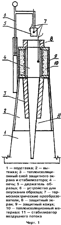
"Чертеж 1"
