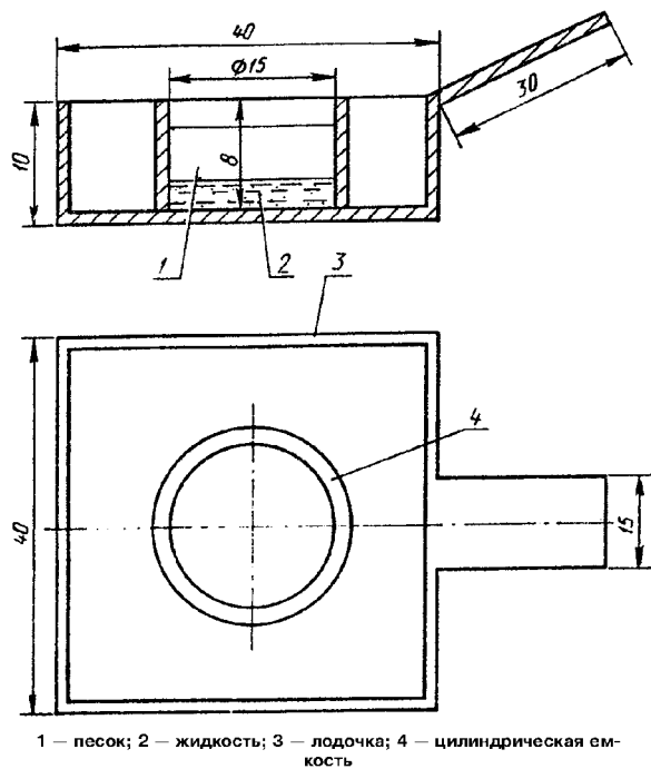
Черт. 24
