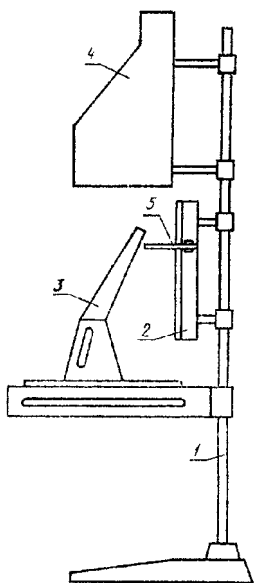
1 – стойка; 2 – электрическая радиационная панель; 3 – рамка держателя образца; 4 – вытяжной зонт; 5 – запальная горелка
