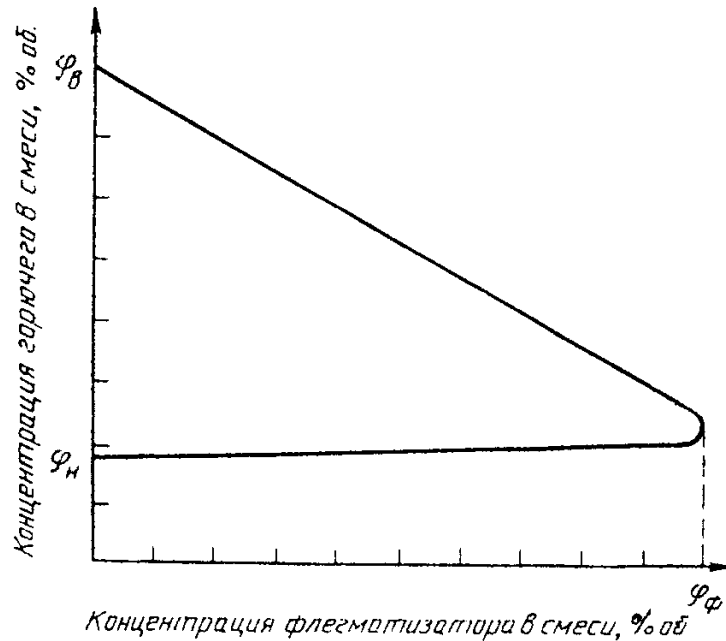
Черт. 21
