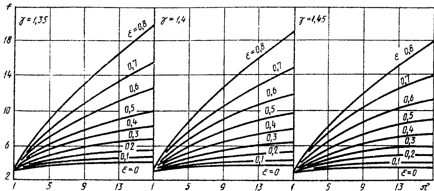
"Чертеж 26"
