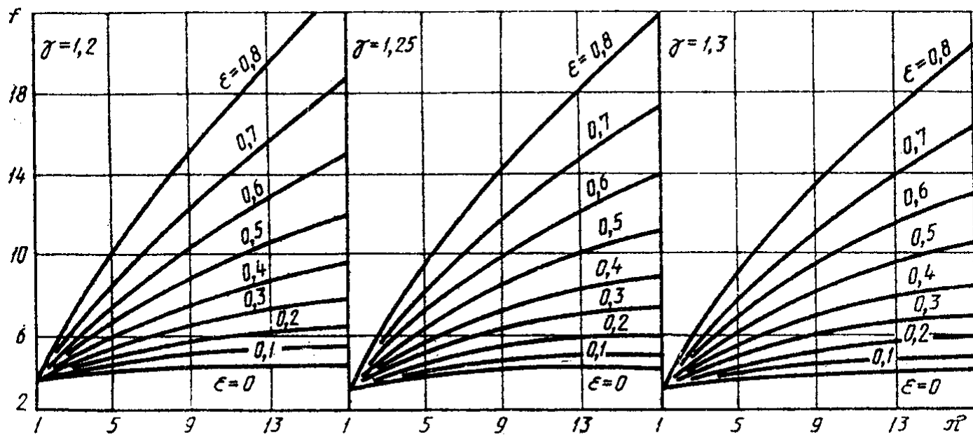
Черт. 26
