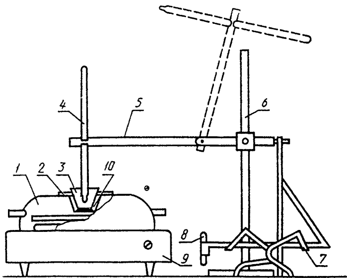
1 — нагревательная ванна; 2 — кольцо из паронита; 3 — фарфоровый тигель; 4 — термометр; 5 — держатель термометра; 6 — штатив; 7 — подставка для горелки; 8 — газовая горелка; 9 — нагревательное устройство; 10 — асбестовая прокладка
