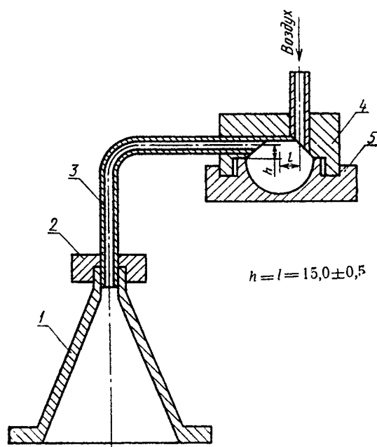
1 — конус; 2 - гайка накидная; 3 — патрубок; 4 — корпус форкамеры; 5 — доньшко
