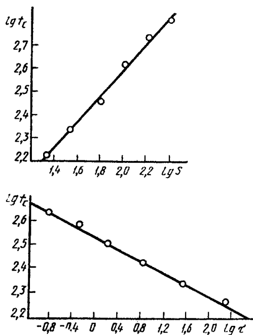
Черт. 29
