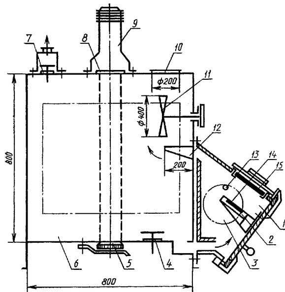
1 — камера сгорания; 2 — держатель образца; 3 — окно из кварцевого стекла; 4, 7 — клапаны продувки; 5 — приемник света; 6 — камера измерений; 8 — кварцевое стекло; 9 — источник света; 10 — предохранительная мембрана; 11 — вентилятор; 12 — направляющий козырек; 13 — запальная горелка; 14 — вкладыш; 15 — электронагревательная панель
