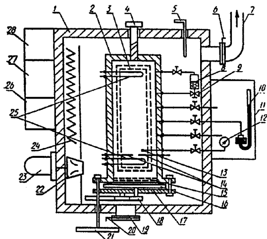
1 — термошкаф; 2 — реакционный сосуд; 3 — смотровое окно; 4 — продувочные патрубок; 5 — термоэлектротрансформатор блока регулирования температуры; 6 — задвижка; 7 — вентиляционный патрубок; 8 — испаритель; 9 — вентиль; 10 — ртутный манометр; 11 — пневмоузел; 12 — газовый термометр; 13 — датчик термометра; 14 — электроды источника зажигания; 15 — огнепреградитель; 16 — нижняя крышка; 17 — коромысло; 18 — шестерни; 19 — продувочное отверстие; 20 — заслонка; 21 — штурвал; 22 — вентилятор; 23 — электродвигатель; 24 — электронагреватель; 25 — перемешиватели; 26 — источник зажигания; 27 — электроузел; 28 — блок регулирования температуры
