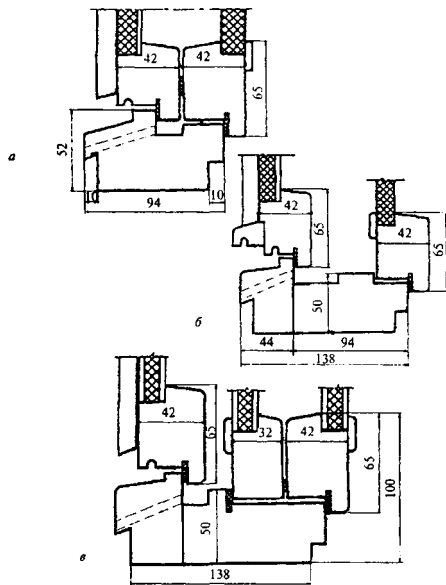
a – заполнение наружного полотна – обшивка, рубероид, мягкая и твердая плиты ДВП, заполнение внутреннего полотна – шлифованная плита ДСП, б – заполнение наружного полотна – аналогично a , заполнение внутреннего полотна – твердые и мягкие плиты ДВП, в – заполнение наружного полотна – полостоякая фанера толщиной 8 мм, заполнение других полотен – трехслойная сэндвич-панель с пеноутеплителем
