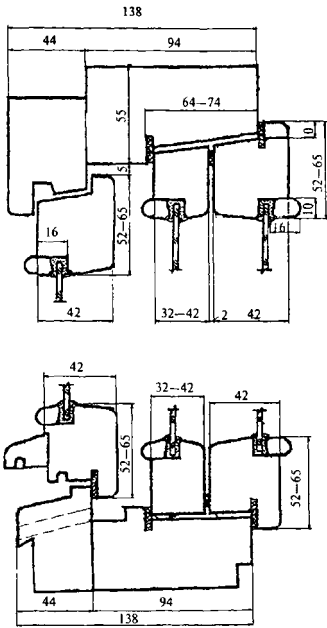
Рисунок 5 – Примеры конструктивных решений оконных блоков раздельно-спаренной конструкции
