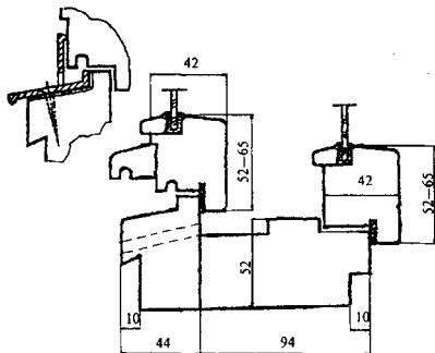
Рисунок 4 – Примеры конструктивных решений оконных блоков раздельной конструкции
