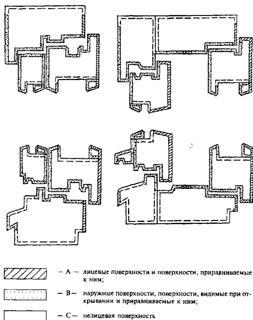
Рисунок 11 – Примеры определения видов поверхностей деталей
