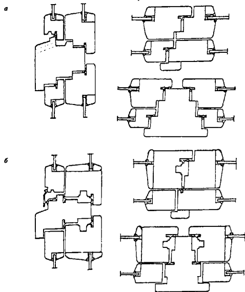
Рисунок 2 – Примеры конструктивных решений оконных блоков спаренной конструкции на базе коробки по ГОСТ 24700 (импостные и безимпостные притворы)
