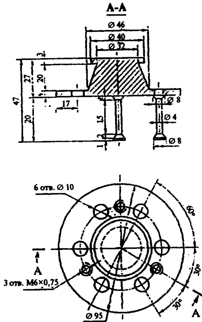
Рисунок 3 — Прибор Красного
